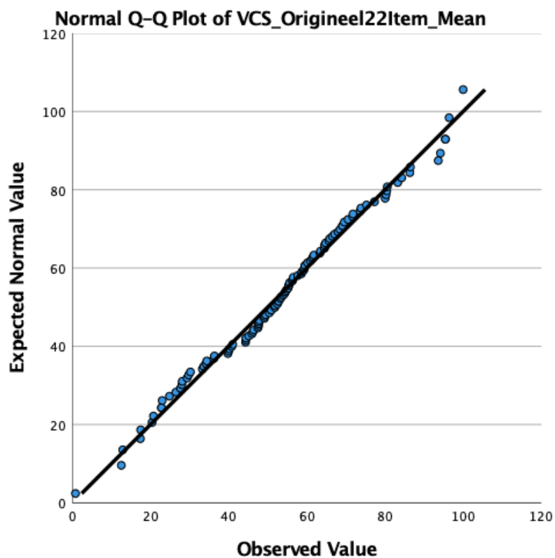
Figuur 1. Q-Q plot van de scores van de afhankelijke variabele
